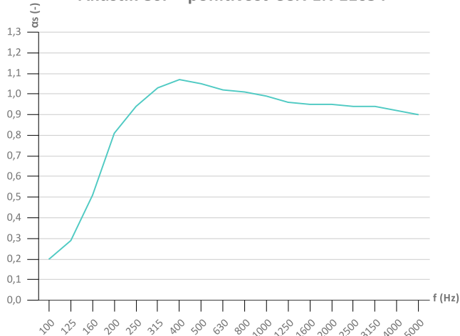
Akustik 80P - pohltivost ČSN EN 11654
