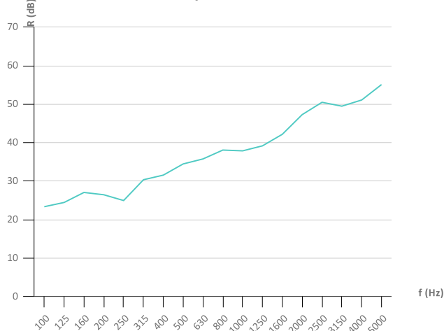
Akustik 80P - neprůzvučnost - EN ISO 10140-2
