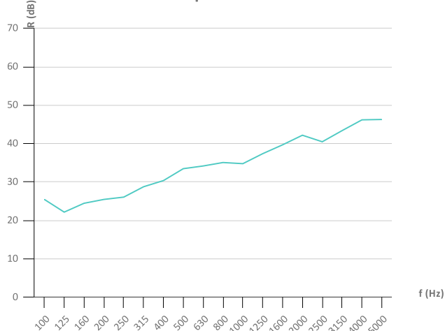
Akustik 40P - neprůzvučnost - EN ISO 10140-2
