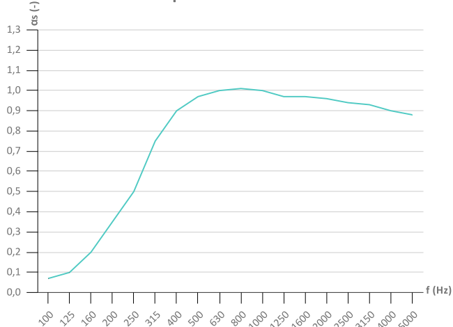
Akustik 40P - pohltivost - ČSN EN 11654
