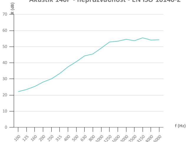
Akustik 140P - neprůzvučnost - EN ISO 10140-2
