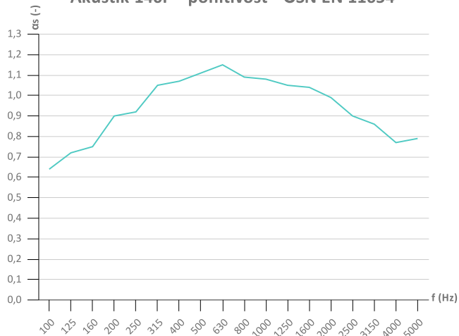
Akustik 140P - pohltivost - ČSN EN 11654
