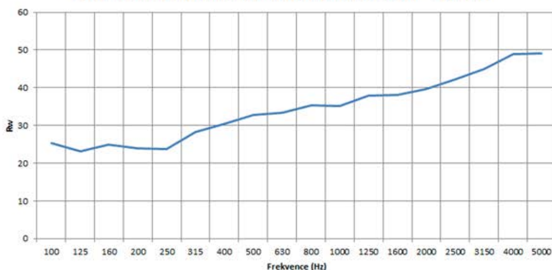
Graf laboratorní vzduchové neprůzvučnosti R_w = 35,3 dB
