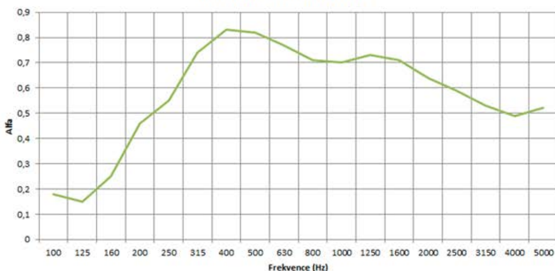
Graf činitele pohltivosti
