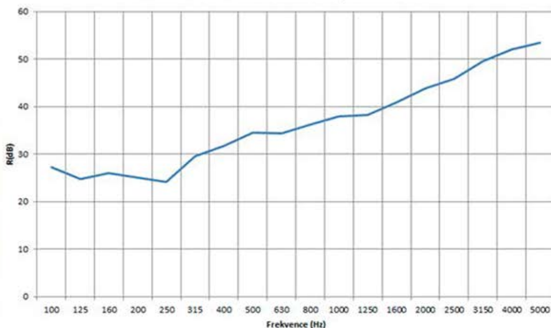
Graf laboratorní vzduchové neprůzvučnosti
