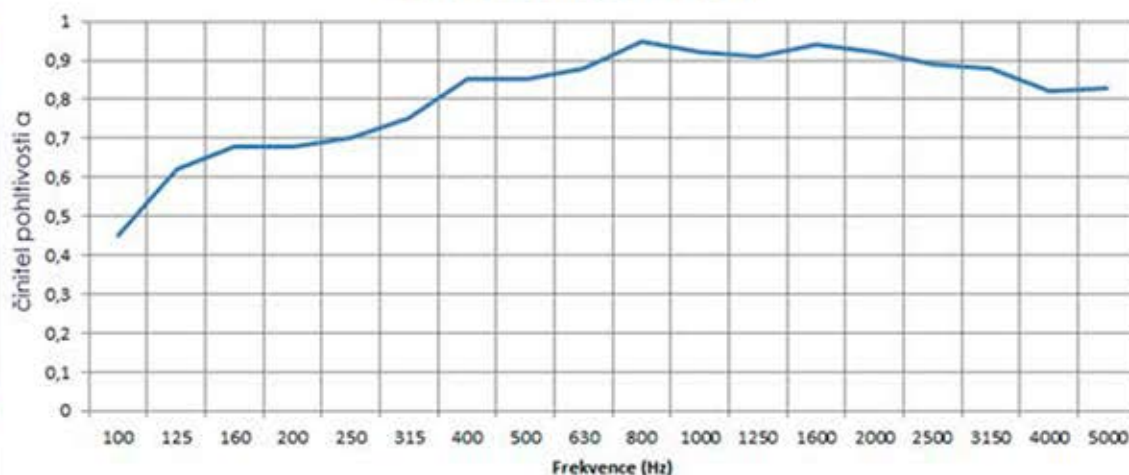
Graf činitele pohltivosti
